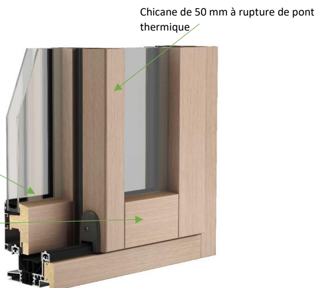
Coupe intérieure bois
